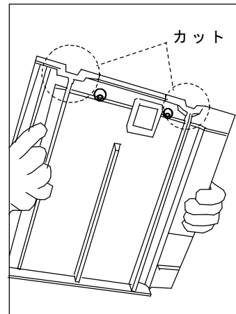
3. 瓦の裏の尻剣をカットします。
