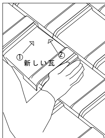
7. ①最初に瓦を上方向に差し込んで下さい（矢印方向） ②次に瓦を右へずらしアンダーラップを差し込んで下さい（矢印方向）
