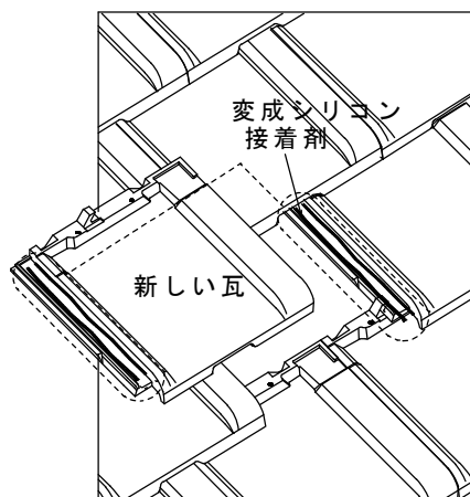
4. 変成シリコン接着剤を塗布します。
