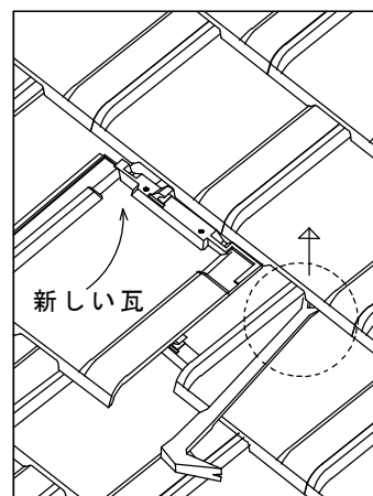
6. 左上の隣の瓦を持ち上げ、差替え用瓦を挿入します。
