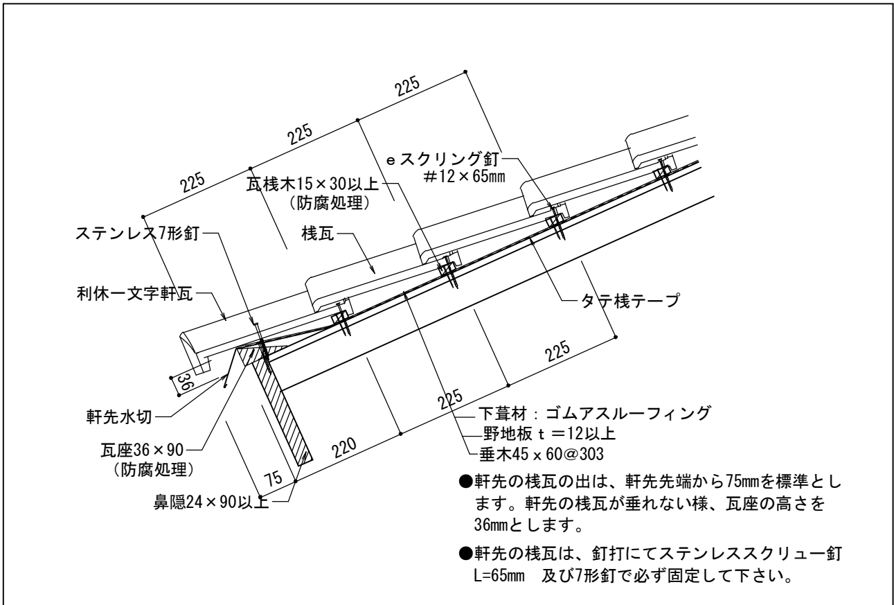
【軒先の納まり】
