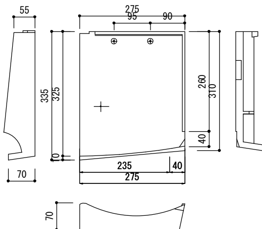
利休一文字角瓦 (左)
