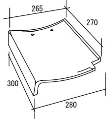
輪型雪止瓦
