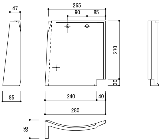
利休一文字袖瓦 (左)
