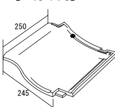
小幅棧瓦 【七分平瓦】
