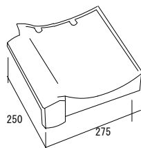
一文字軒瓦 【一文字すりあわせ唐草】
