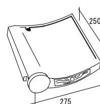
雀口付万十唐草袖角瓦 (左) 【面戸付小角】
