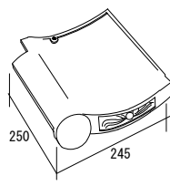
紐袖瓦 (右) 【紐付大袖】
