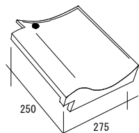
ミノコ棧瓦 (右) 【ミノコ平瓦 (右)】
