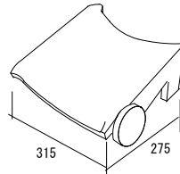
棧瓦片流れ止 (右) 【タレ付大袖】
