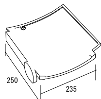
駒一文字袖瓦 (右) 【一文字駒付大袖】
