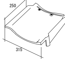
駒一文字袖瓦 (左) 【一文字駒付小袖】
