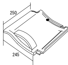
小幅輪型雪止 【七分輪型雪止】
