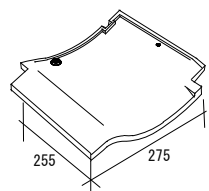
ミノコ棧瓦 (右) 【ミノコ平瓦 (右)】
