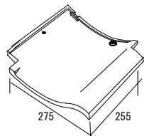
ミノコ棧瓦 (左) 【ミノコ平瓦 (左)】
