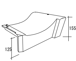
利休一文字袖瓦 (右)
