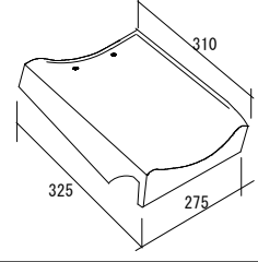
利休一文字角瓦 (左)
