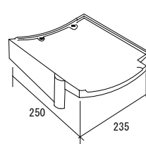
駒一文字袖角瓦 (右) 【一文字駒付大角】
