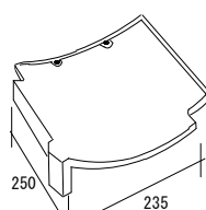
一文字軒瓦 【一文字すりあわせ唐草】
