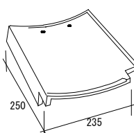
ミノコ万十唐草 (右) 【ミノコ唐草 (右)】
