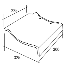
利休一文字袖瓦 (右)
