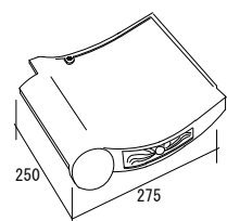
万十袖瓦 (右) 【万十大袖】
