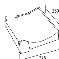
一文字軒瓦 【一文字すりあわせ唐草】
